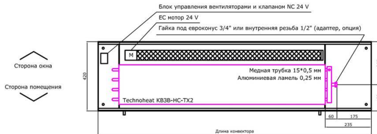
Размеры КВЗВ-НС-ТХ2 - 420х150х....
