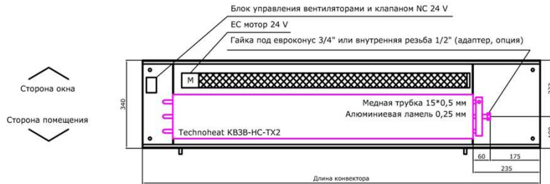
Размеры КВЗВ-НС-ТХ2 - 340х150х...
