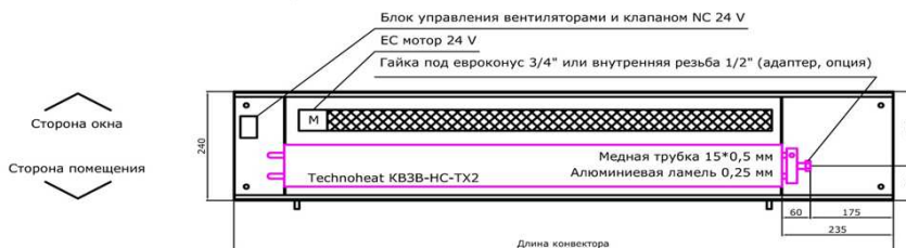
Размеры КВЗВ-НС-ТХ2 - 240x150x....
