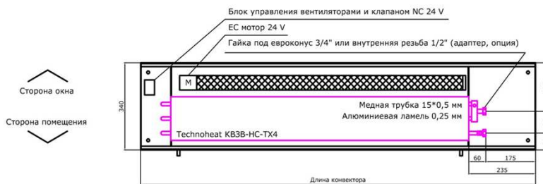
Размеры КВЗВ-НС-ТХ4 - 340х150х...
