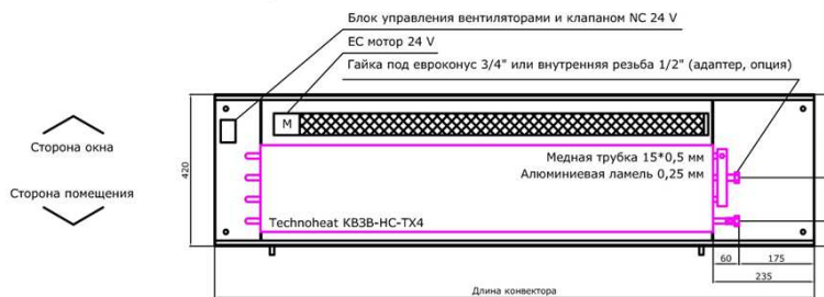
Размеры КВЗВ-НС-ТХ4 - 420х150х....
