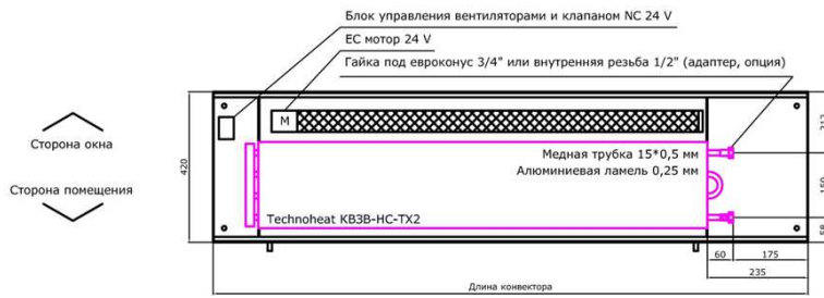
Размеры КВЗВ-НС-ТХ2 - 420х100х....
