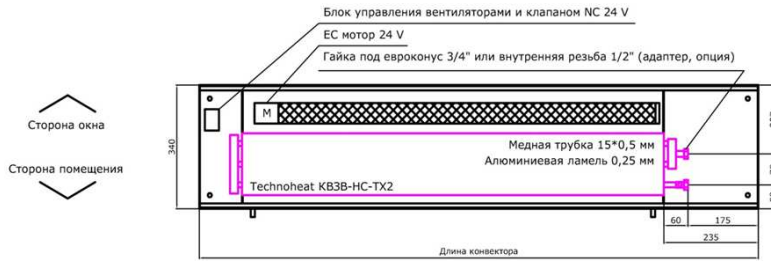
Размеры КВЗВ-НС-ТХ2 - 340х100х...
